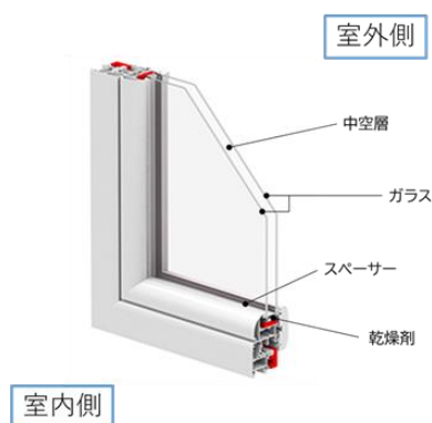
<複層ガラス>
