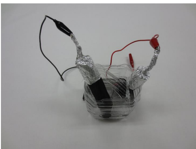
5. ワニ口クリップ付リード線の取り付け
