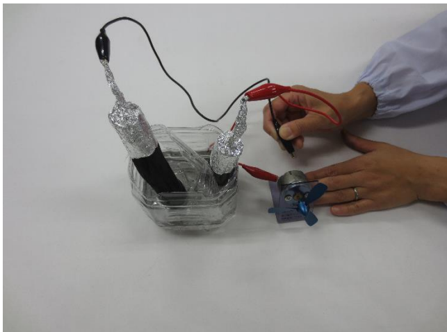
7. プロペラの回転
